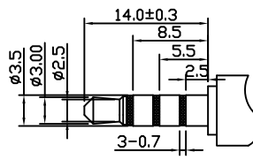
建议插头尺寸
