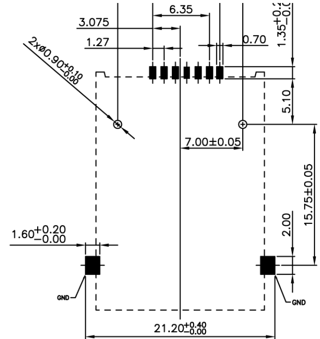
P.C.B LAYOUT
